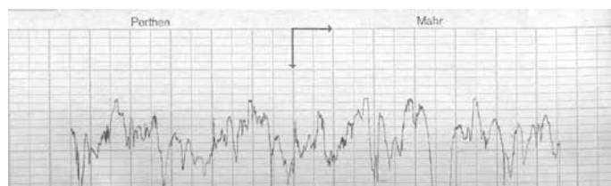
Resultaat na het polijsten met 40 m \mu (blauw).
